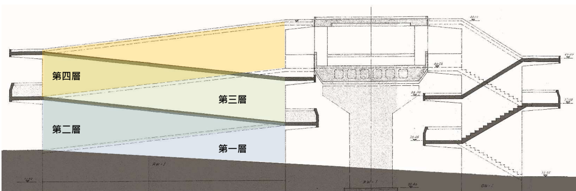
天橋剖面圖
