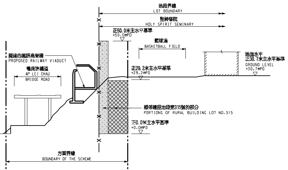
切面圖 SECTION AQ 不按比例 NOT TO SCALE
