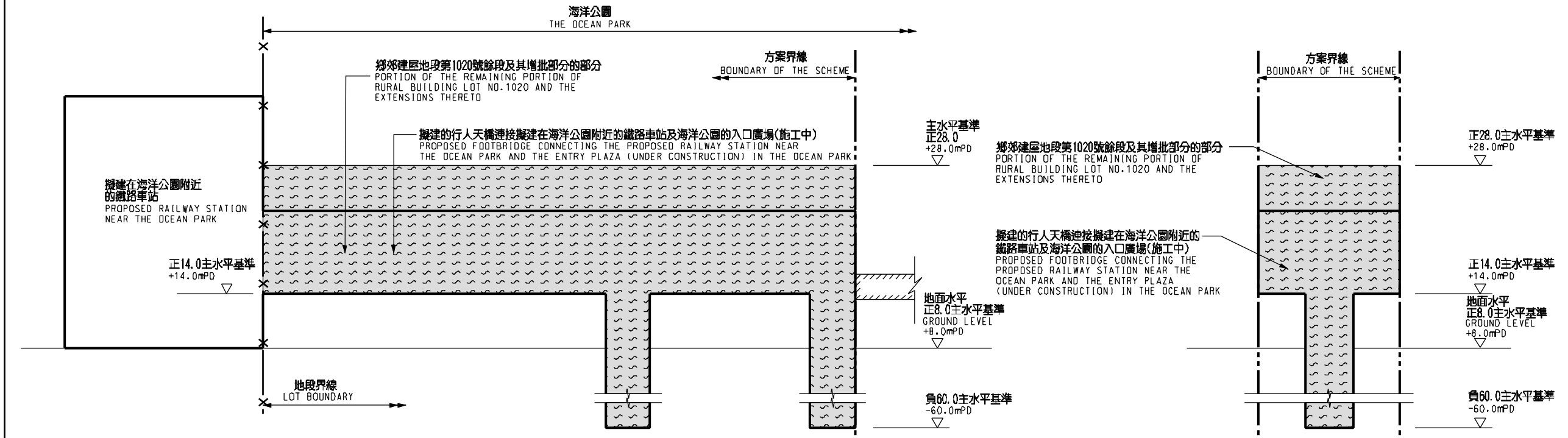
切面圖 SECTION AT 不依比例 NOT TO SCALE
