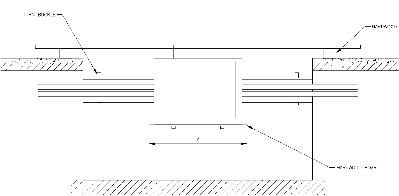
SECTION A-A
