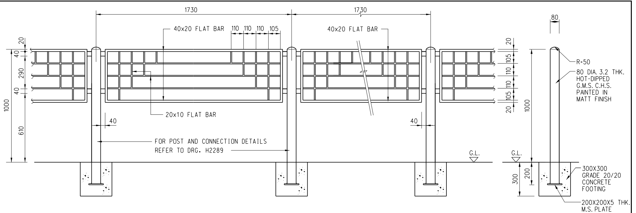
ELEVATION
