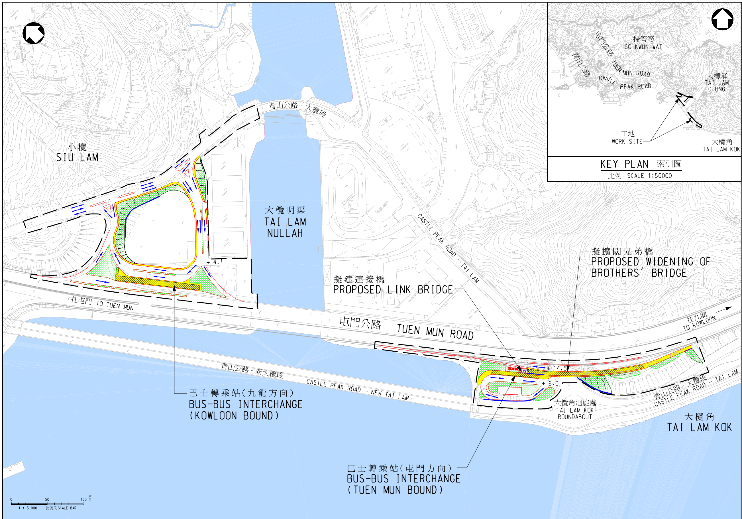
工務計劃項目第76TI號 - 屯門公路巴士轉乘站 - 平面圖 PWP ITEM NO. 76TI - BUS-BUS INTERCHANGES ON TUEN MUN ROAD - LAYOUT PLAN
