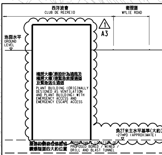
切面圖 SECTION A 不設比例 NOT TO SCALE
