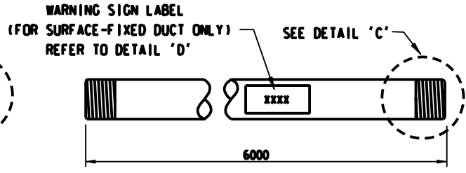
ELEVATION (G.I.)
